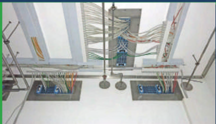
SELLOS ROXTEC
